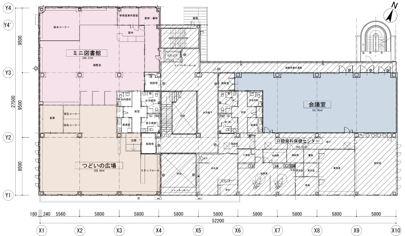
2階平面図
