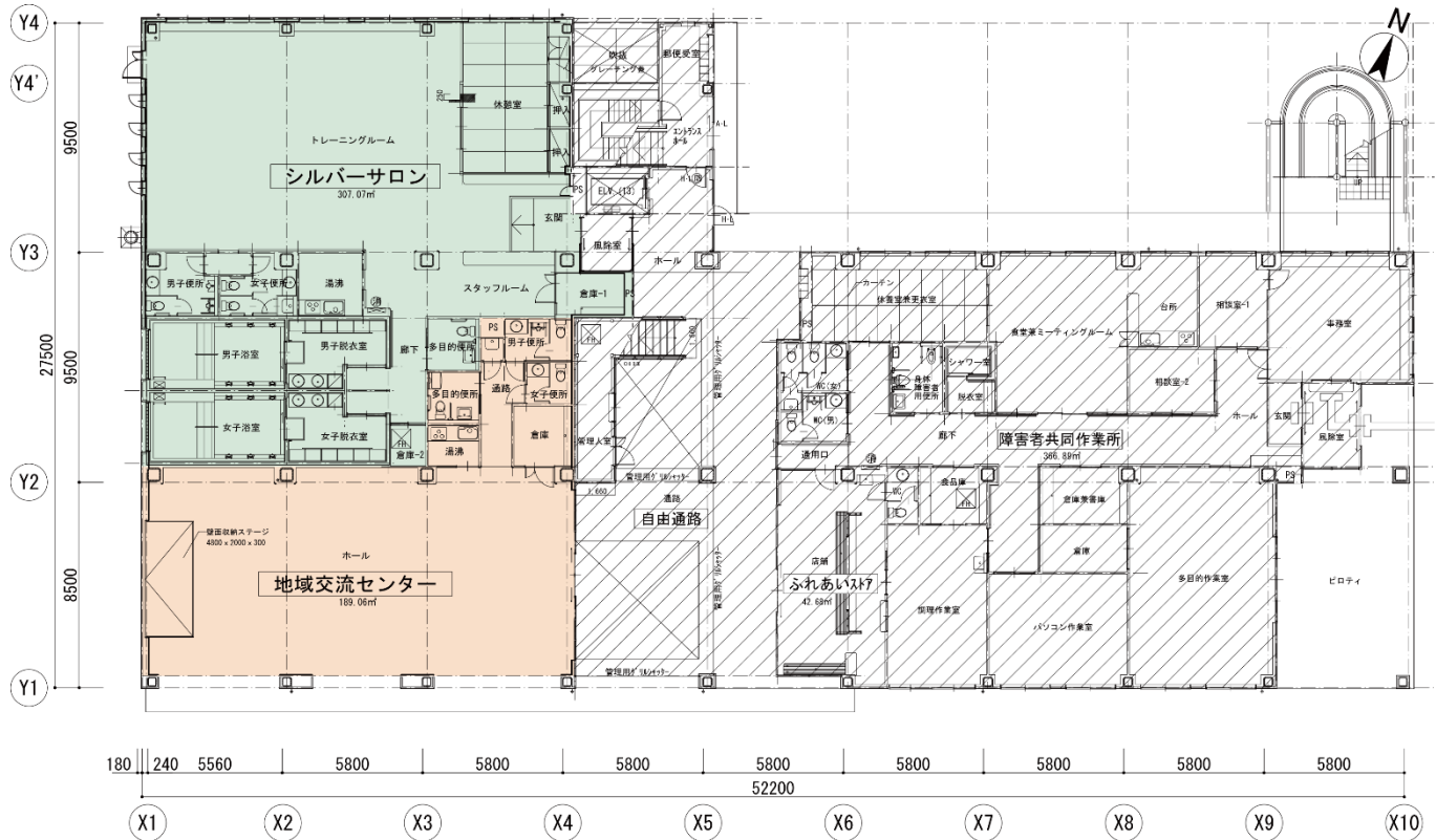
1階平面図
