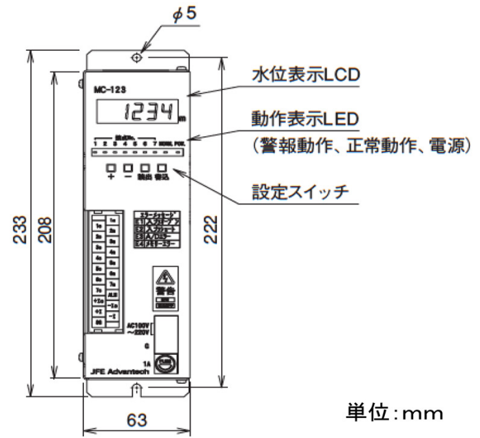
変換器 MC-123型
