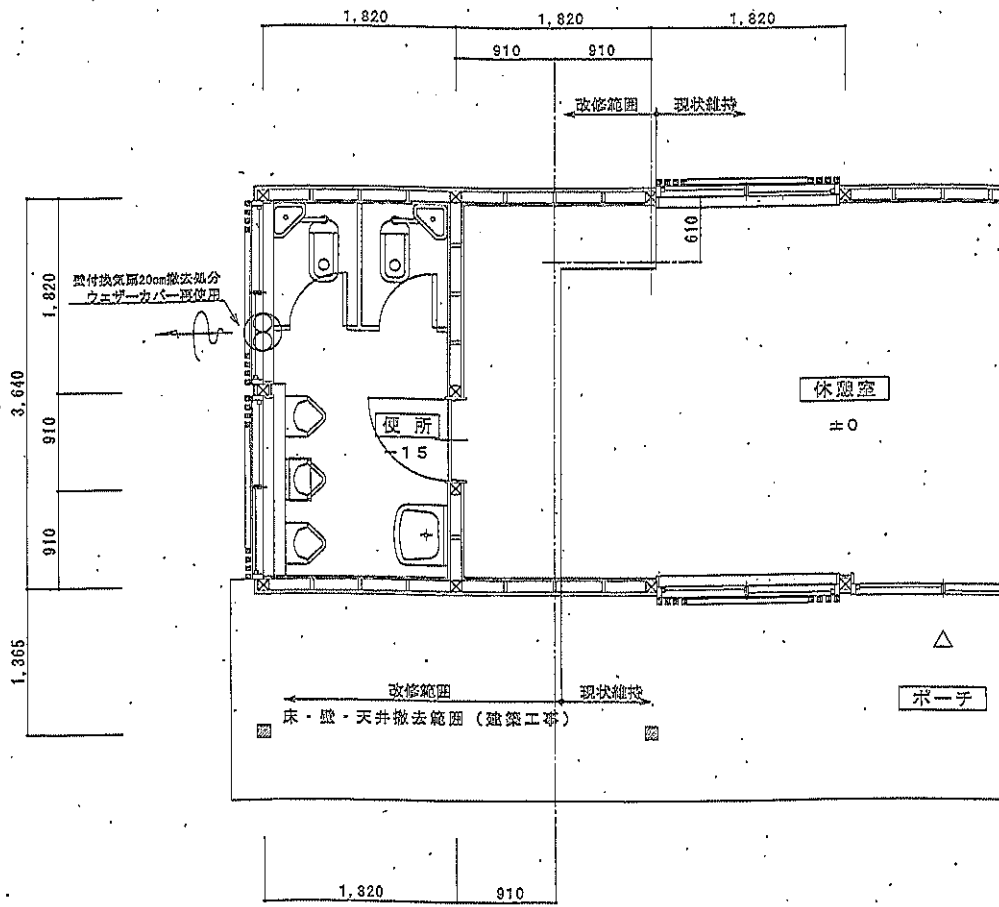
改修前 平面図 S=1/50
