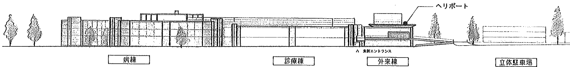
東側立面図 1/1200
