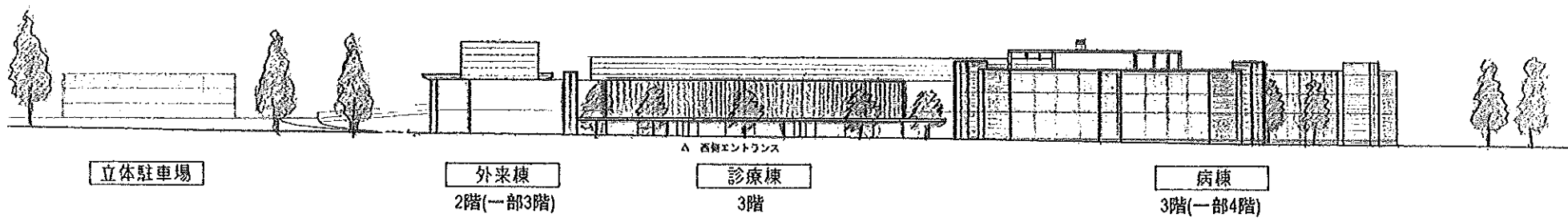
西側立面図 1/1200
