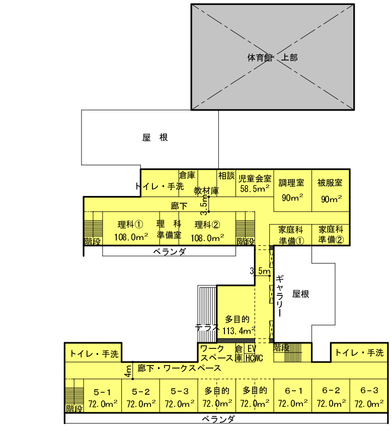
3階床面積 2,422.1m 2 (吹抜除く) 3階平面図
