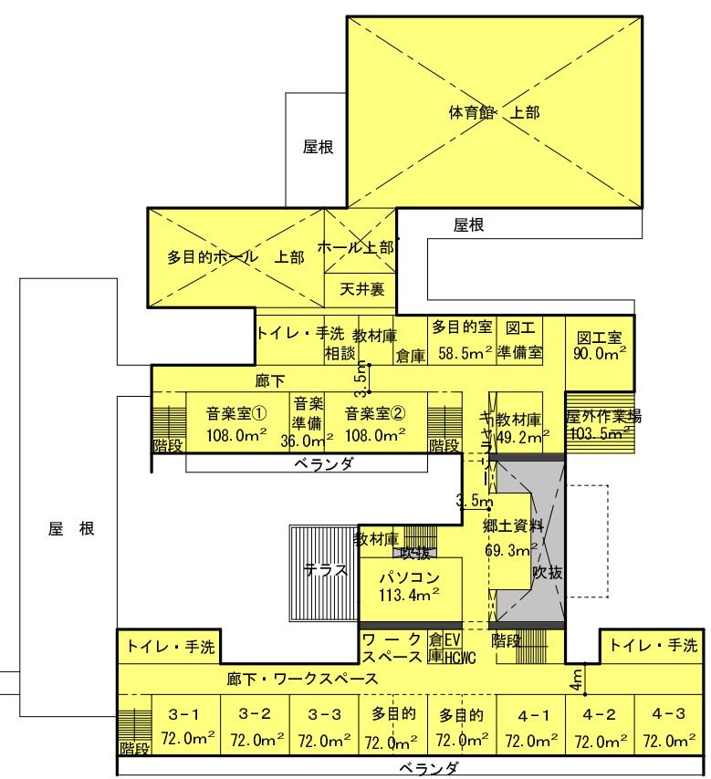
2階床面積 2,549.0m 2 (吹抜除く) 2階平面図
