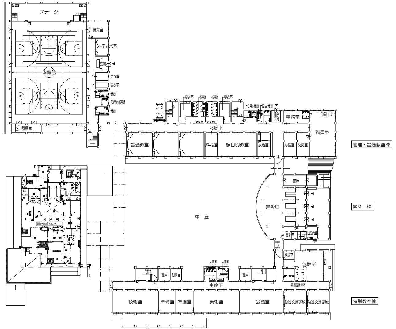
1階平面図
