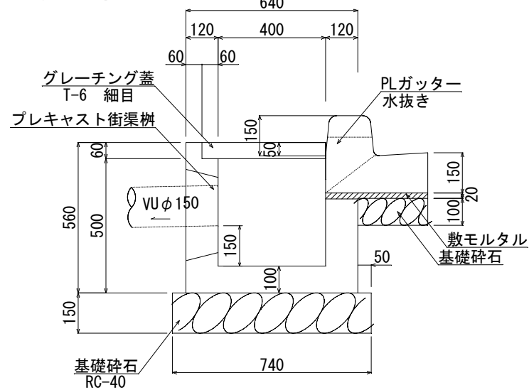
プレキャスト街渠柵 セミフラット対応型
