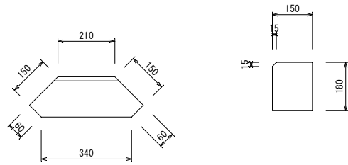
5号コーナー S=1:10
