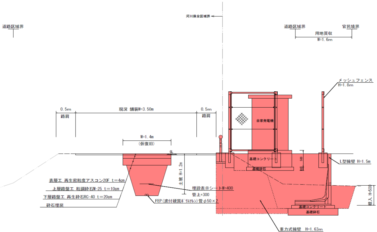
標準断面図
