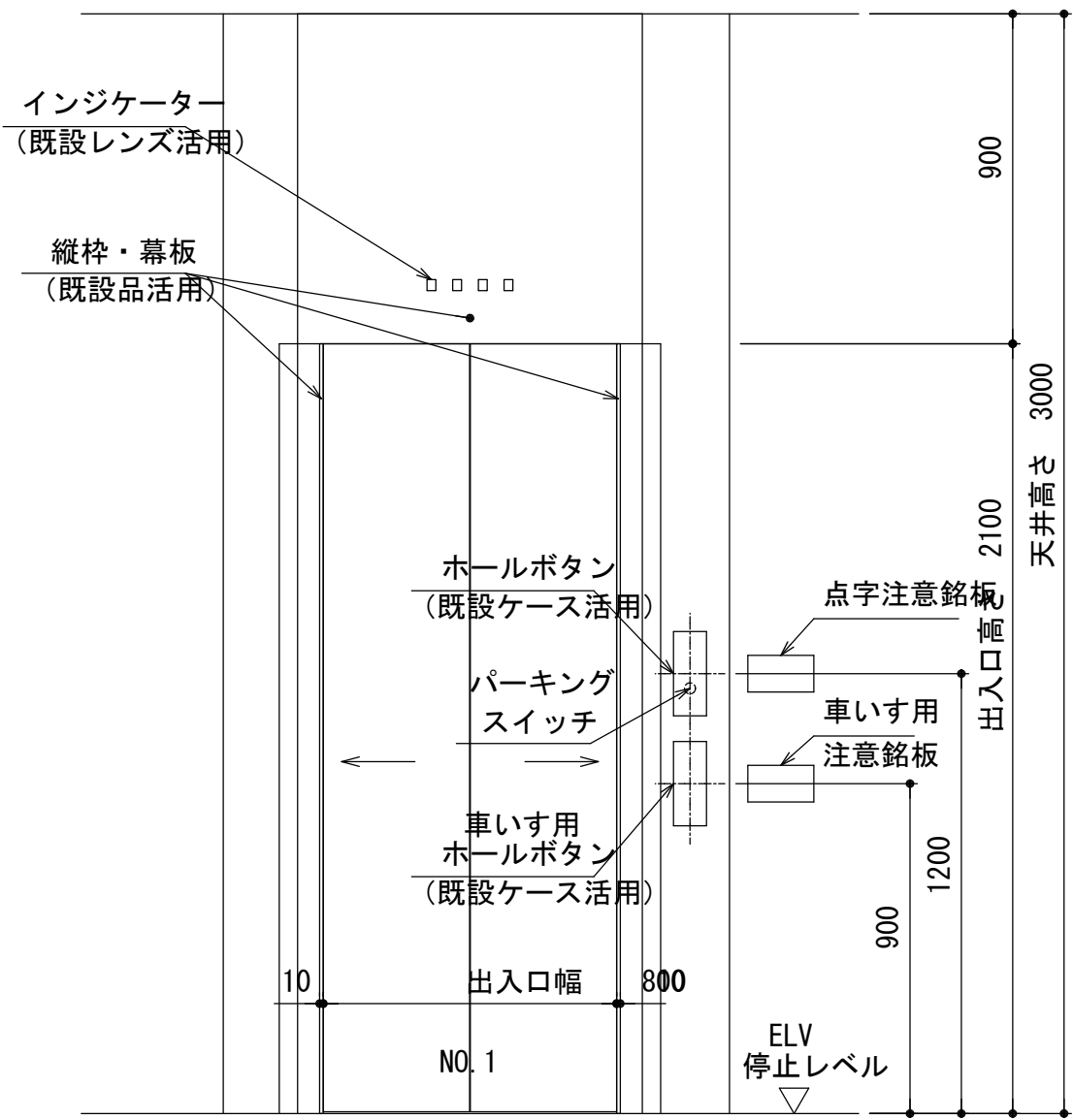
1階 出入口正面及断面図 (1 : 20)
