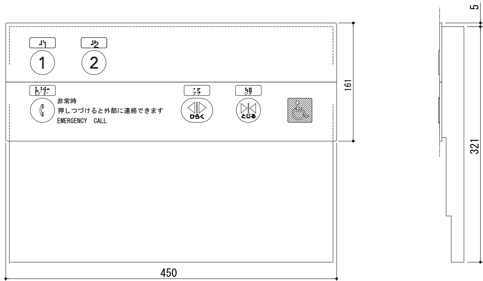
副操作盤（1：3）
