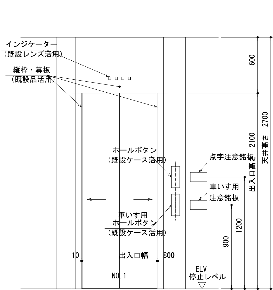
2階 出入口正面及断面図 (1 : 20)
