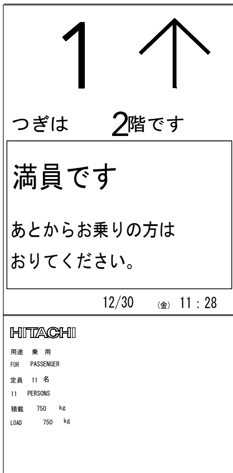
用途銘板及び表示部詳細図 (1:2)
