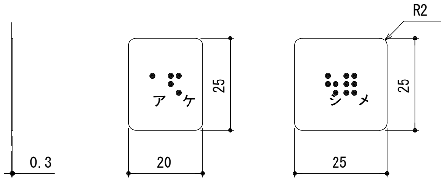
点字銘板意匠(1:1)
