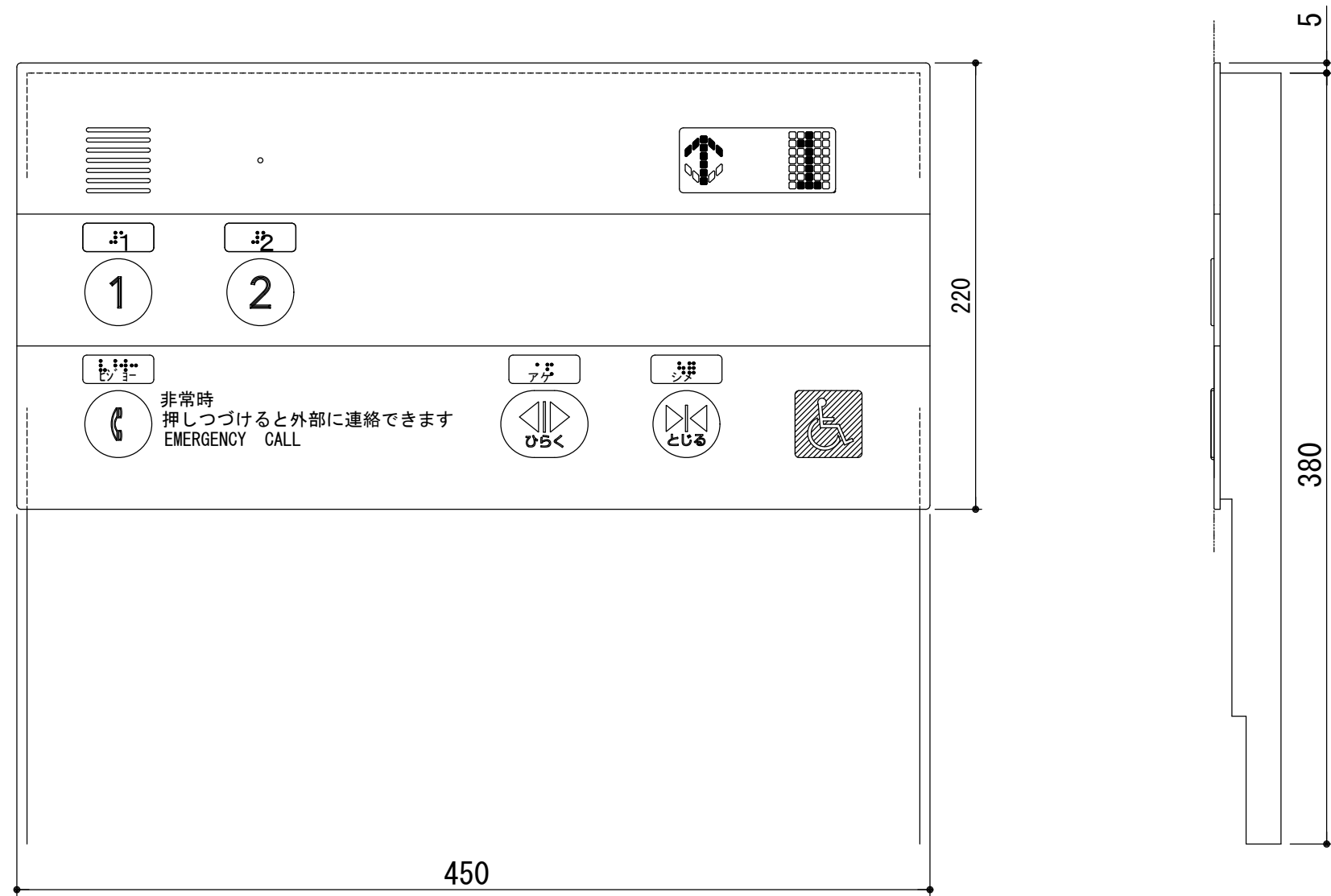
主操作盤（1：3）
