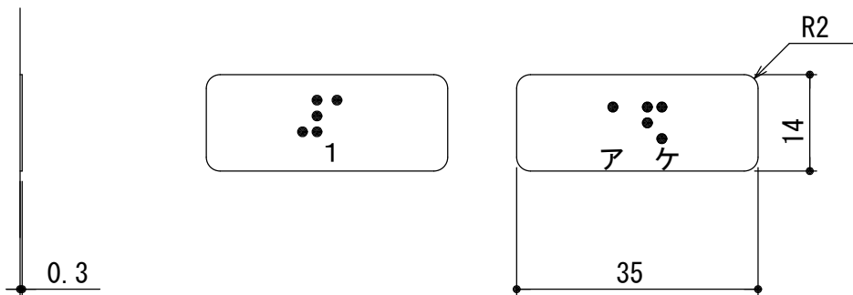
点字銘板意匠（1：1） 注）点字下部の数字、片板名は銘板にはありません。
