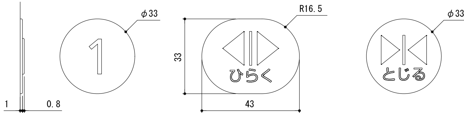
押ボタン意匠 (1:1)
