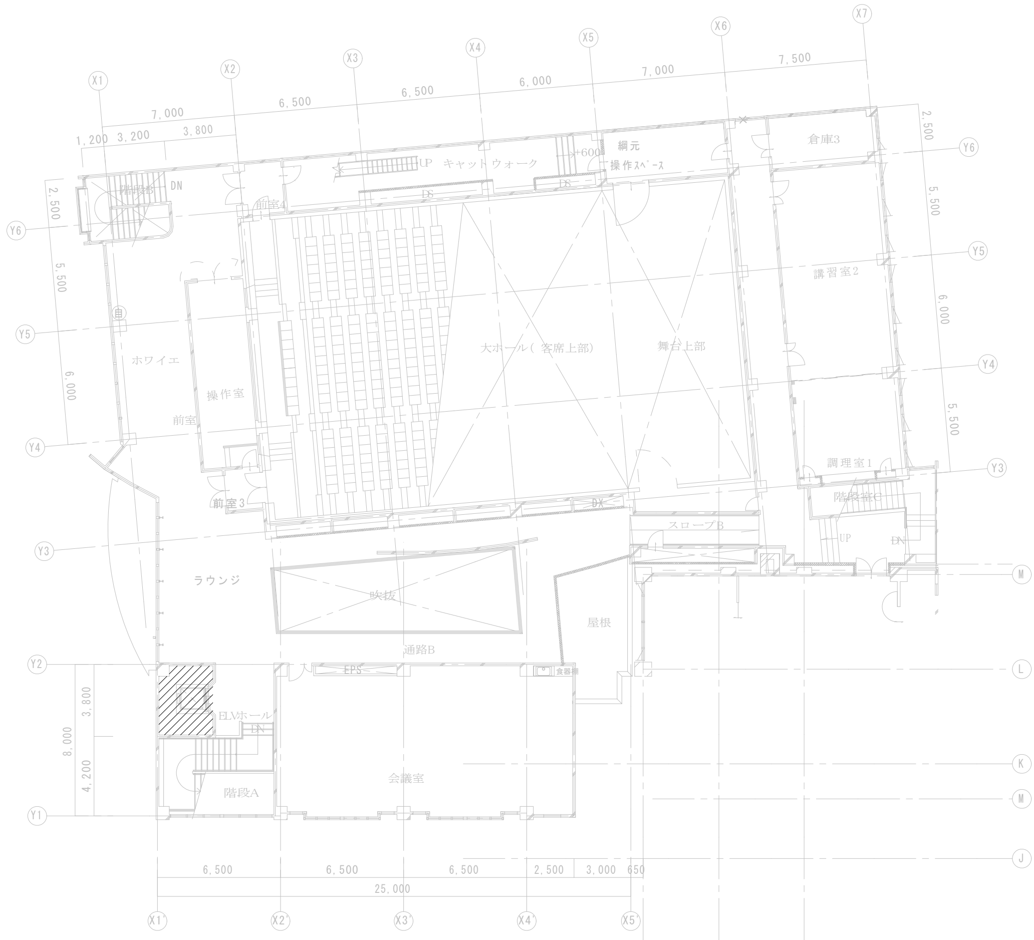
駒の里ふれあいセンター 2階 平面図
