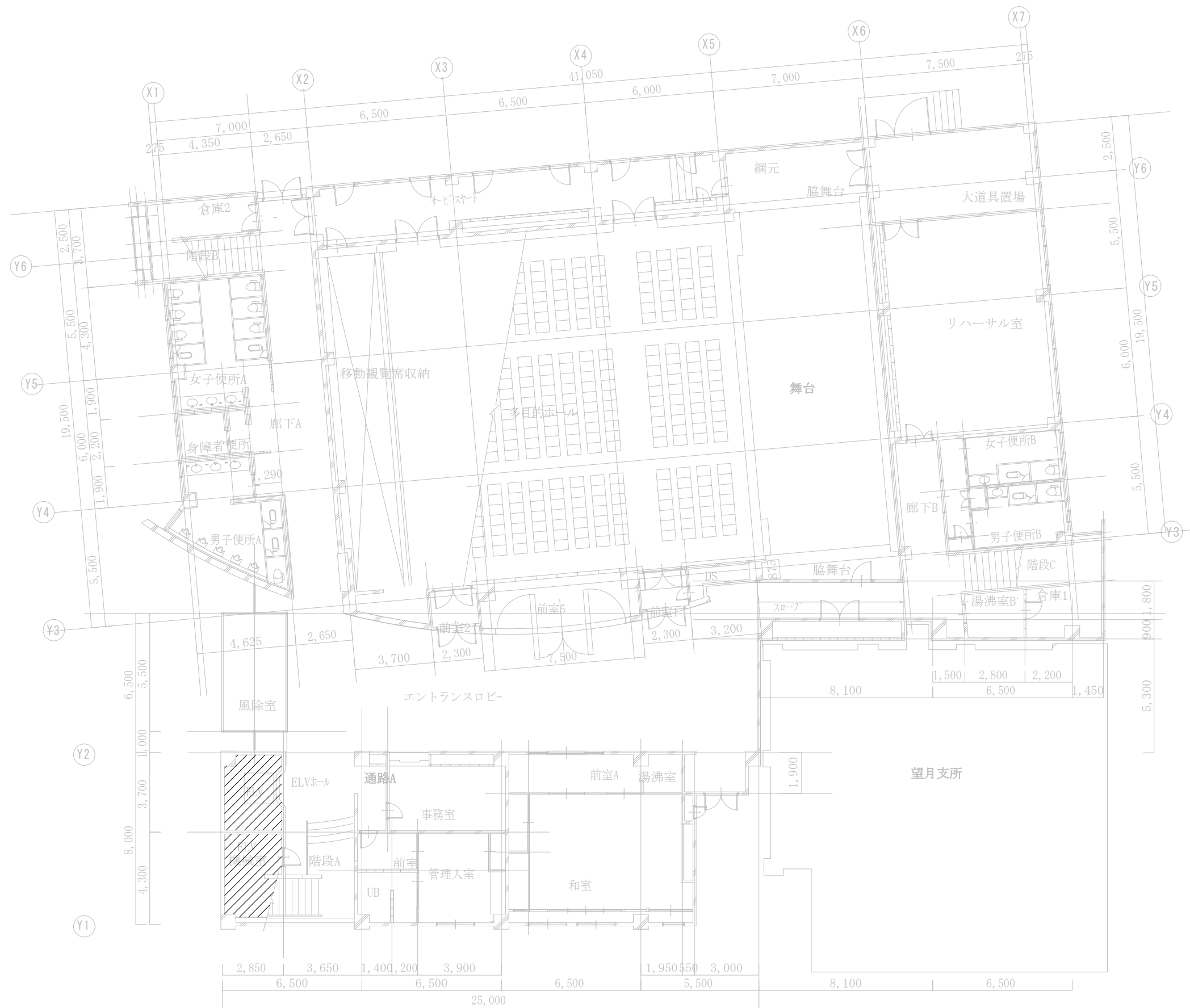
駒の里ふれあいセンター 1階 平面図
