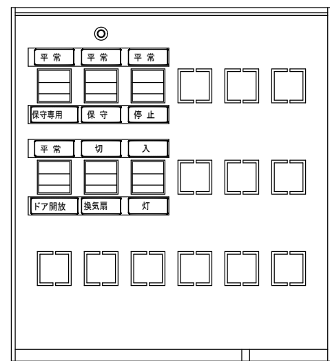
下部スイッチボックス内 (1:2)
