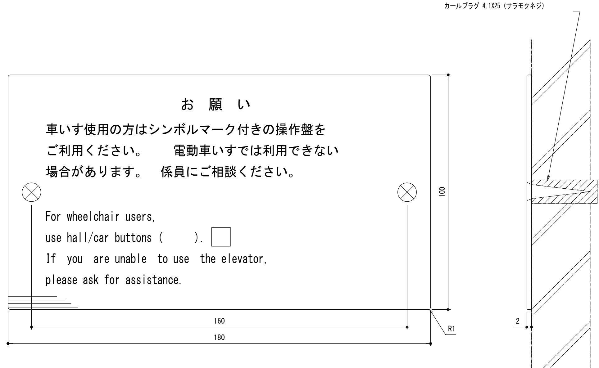
車いす注意銘板意匠図（乗場用）（1：1）
