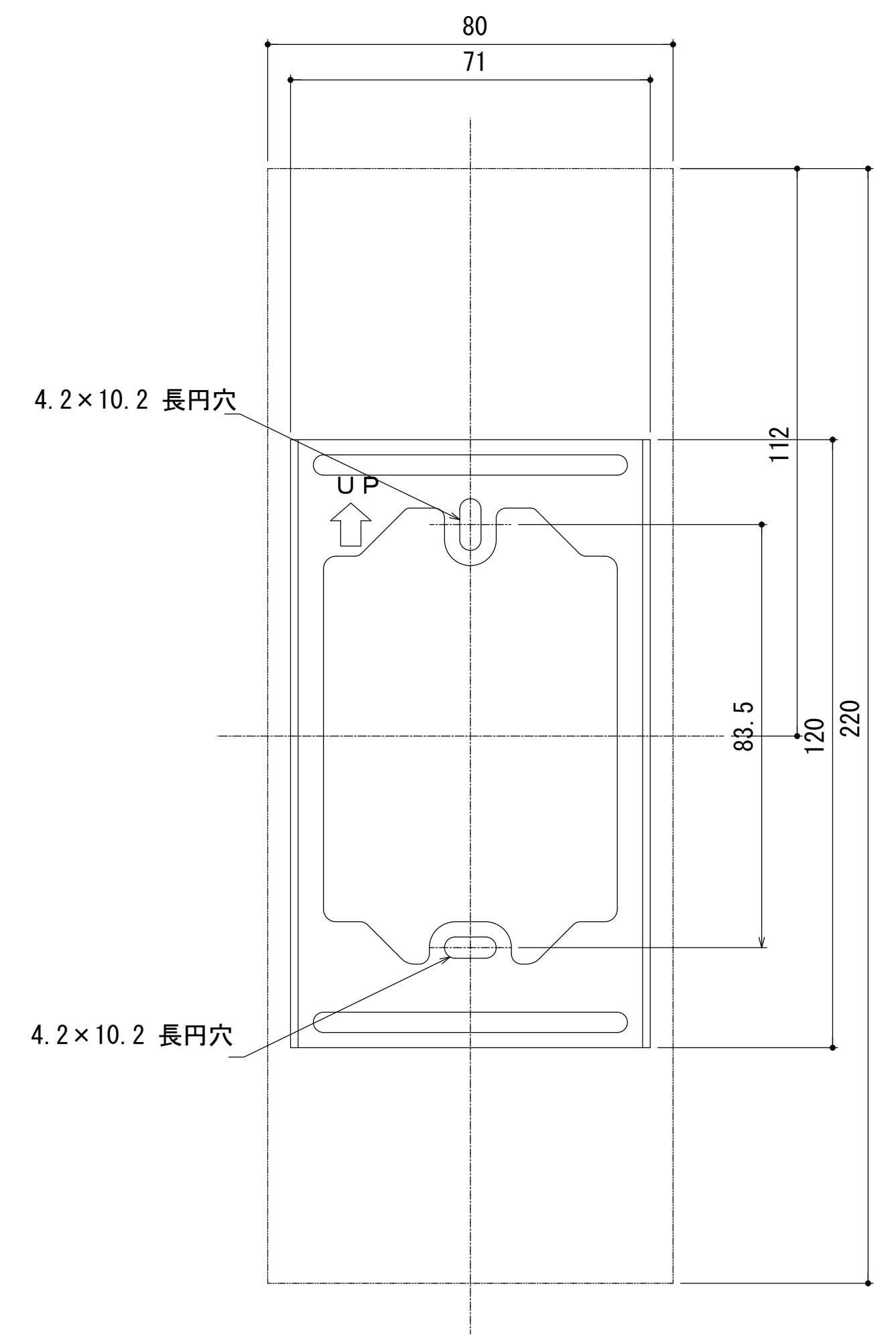
壁取付位置図 ※ 取付はM4ねじにて2箇所止め
