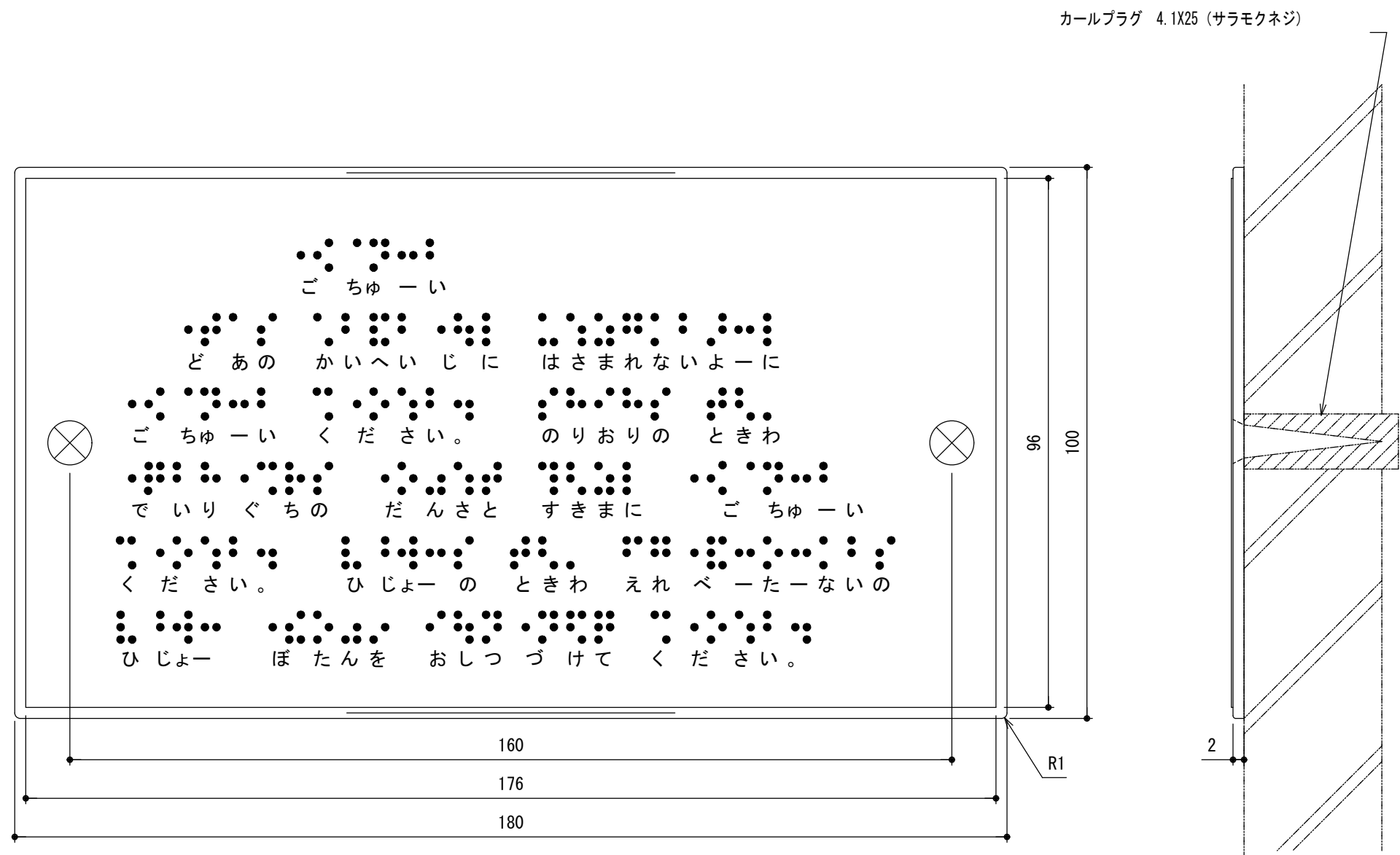
点字注意銘板意匠図（乗場用）（1：1）
