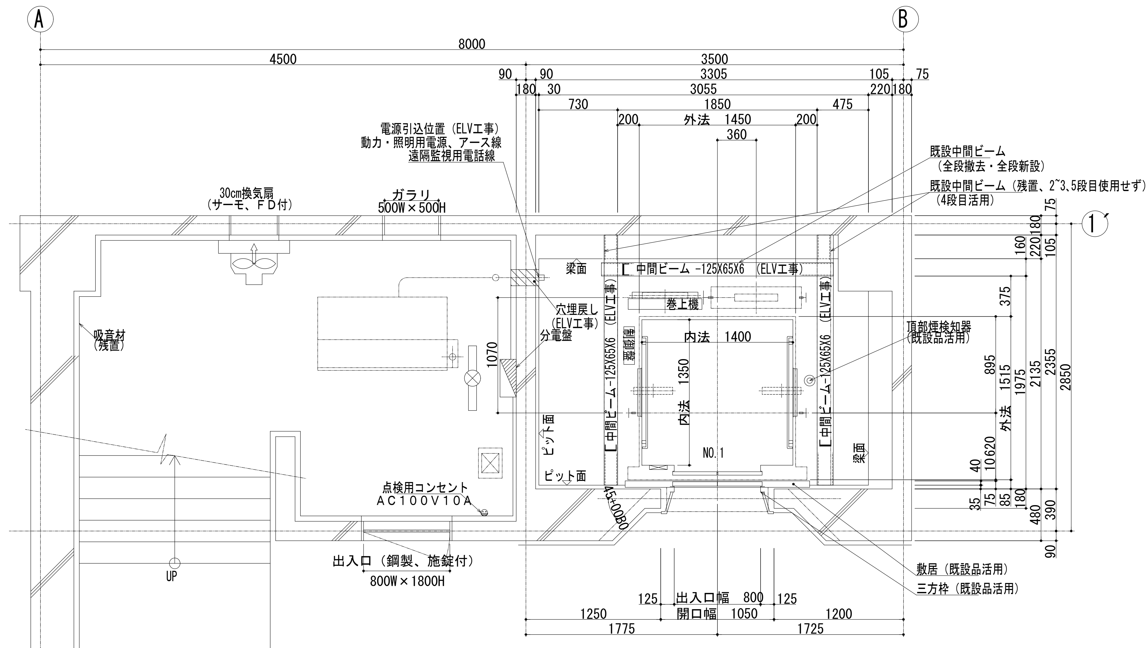
1、2階 昇降路平面図（1：20）
