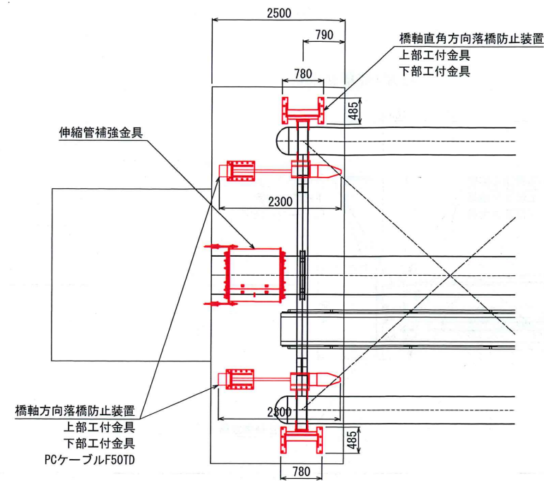
平面図 S=1:50
