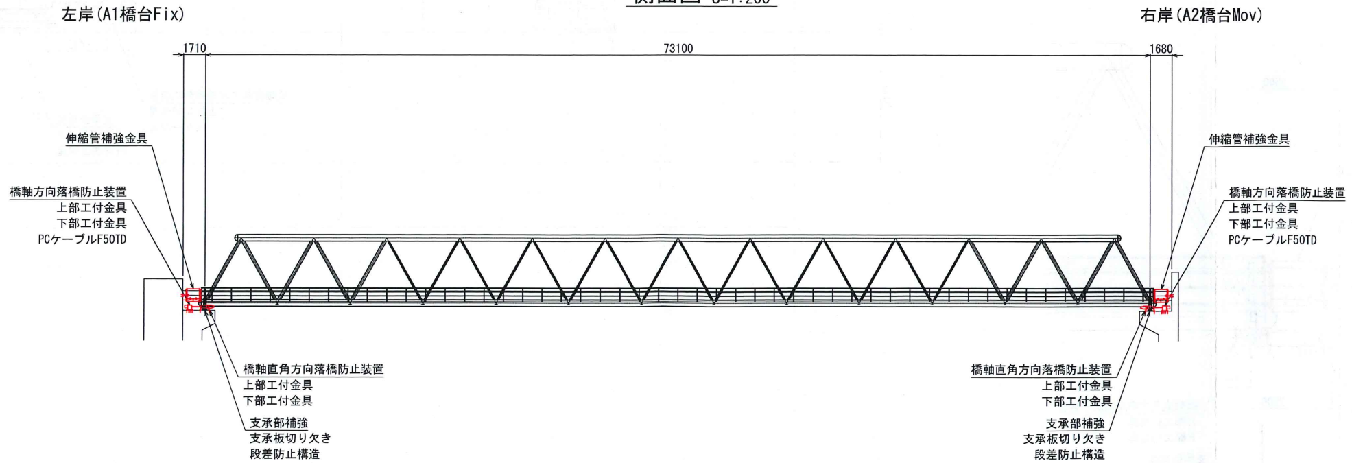
側面図 S=1:200
