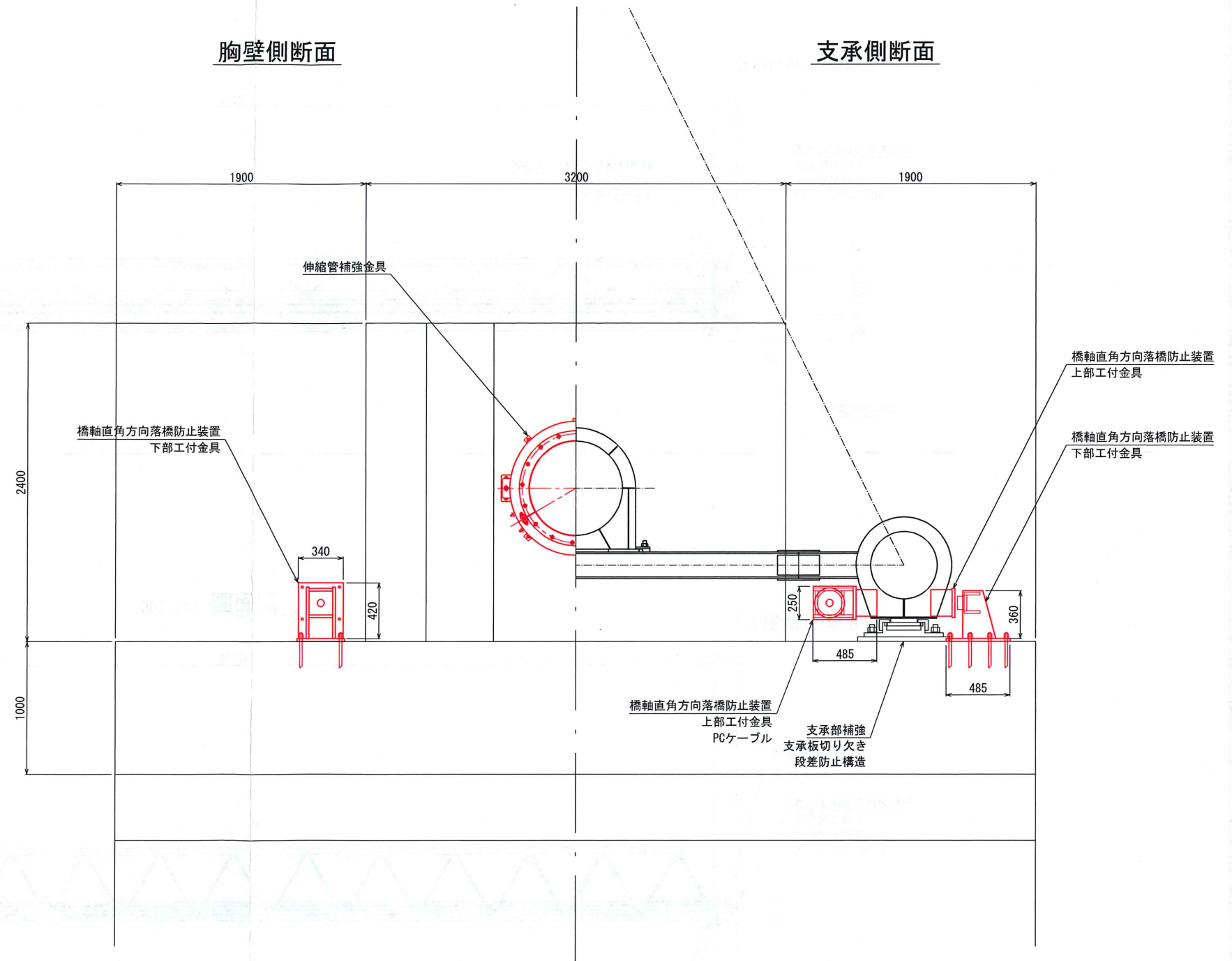
断面図 S=1:20
