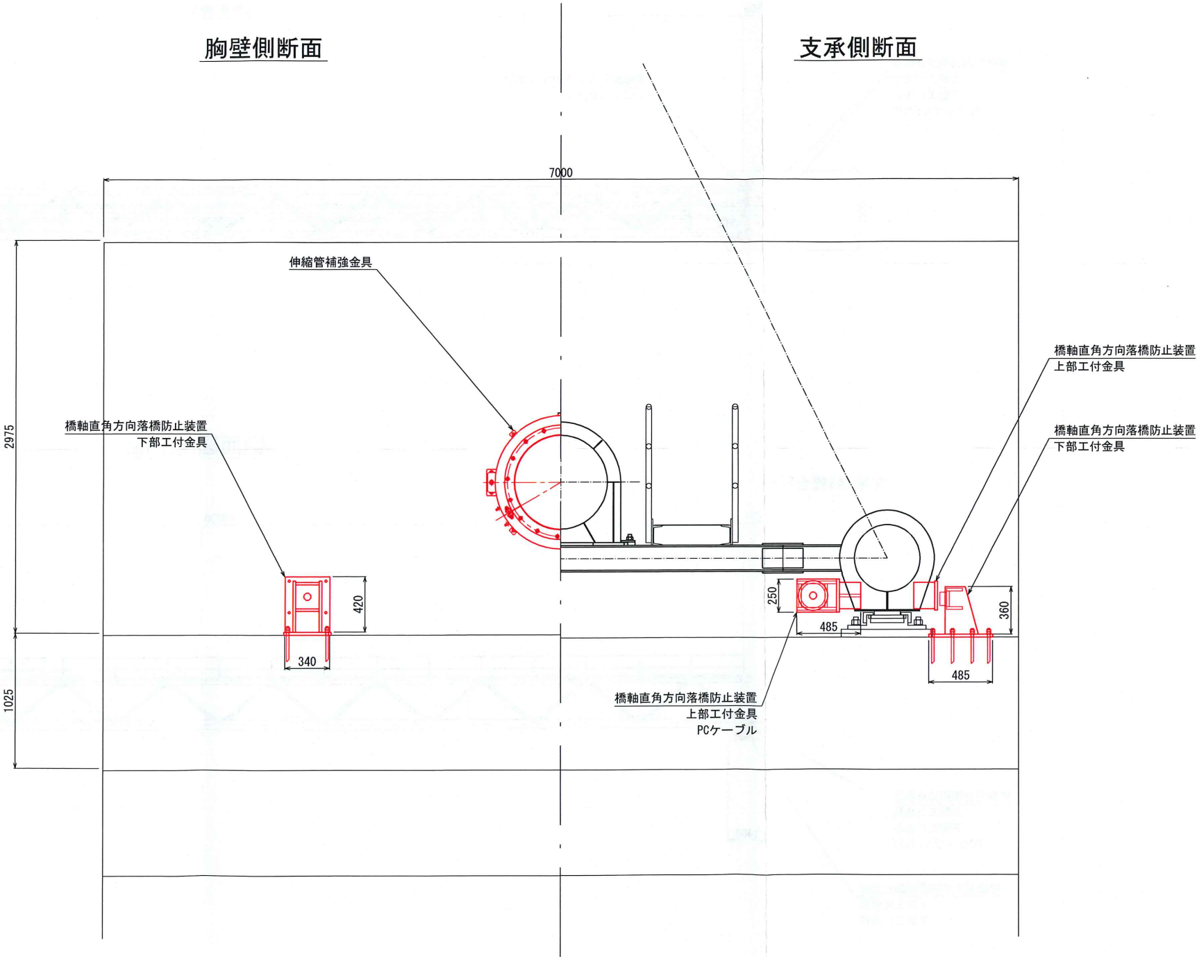
断面図 S=1:20
