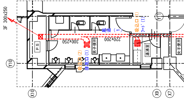
5階 平面図 (WC脱給湯室)
