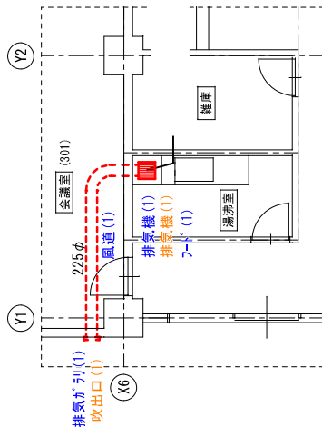
3階平面図 (税務課 給湯室)
