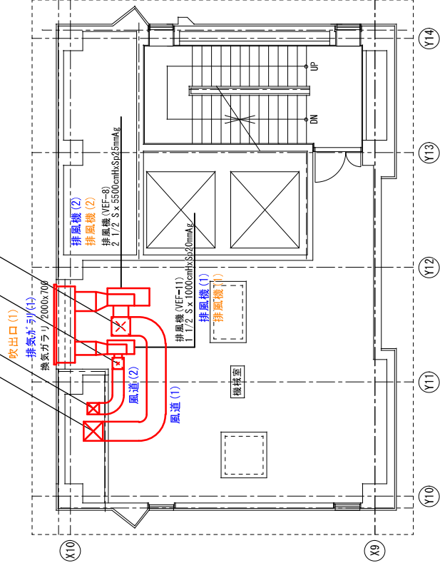
P1階平面図
