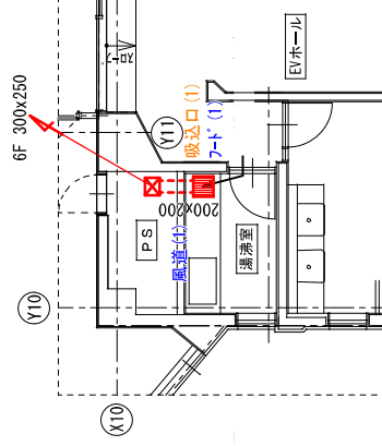
6階 平面図 (WC脱給湯室)
