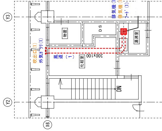
4階 平面図 (市最室 給湯室)
