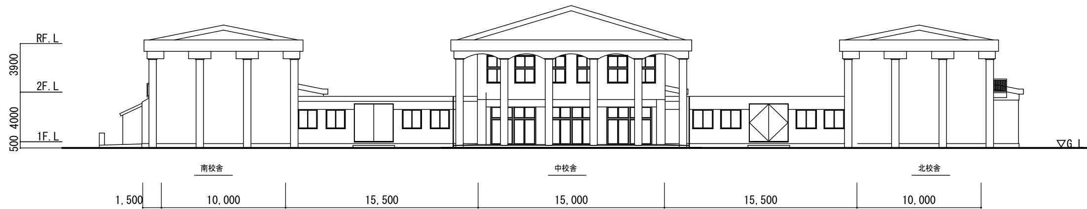
東側立面図
