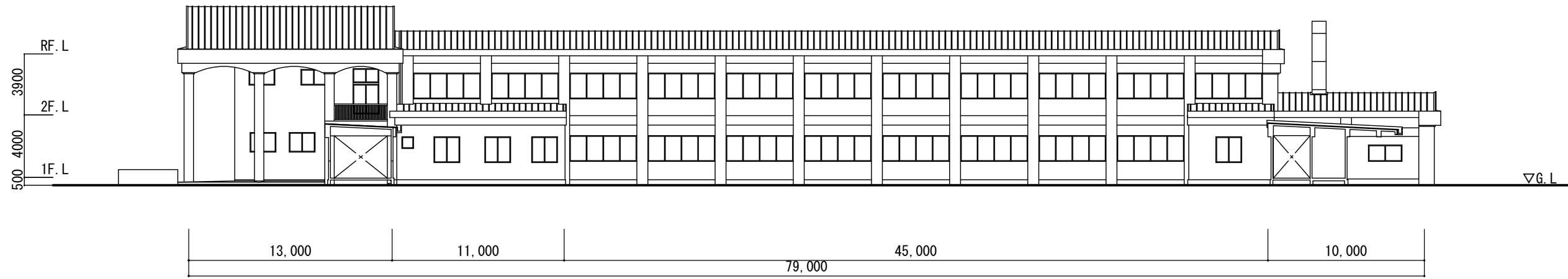
中校舎 北側立面図
