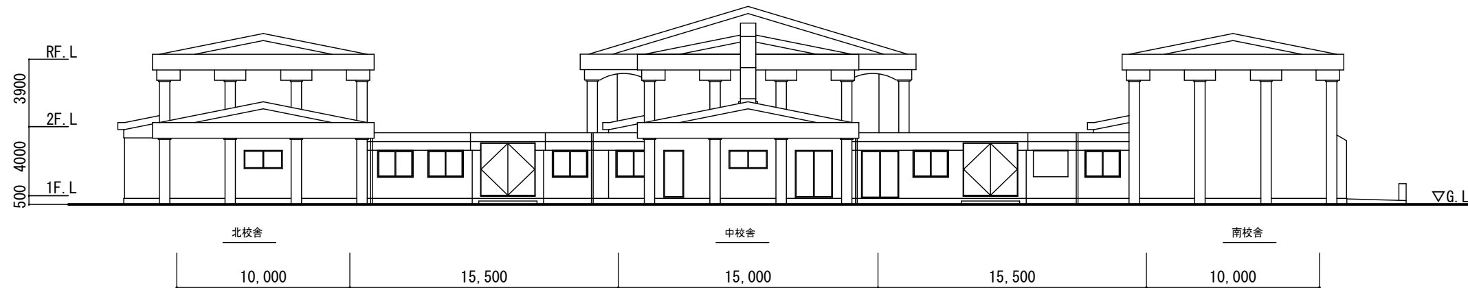
西側立面図
