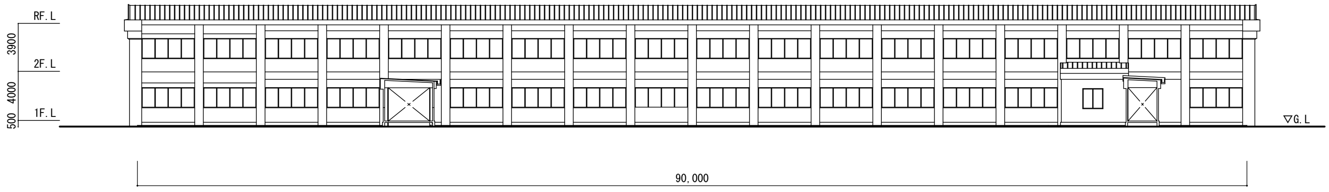
南校舎 北側立面図
