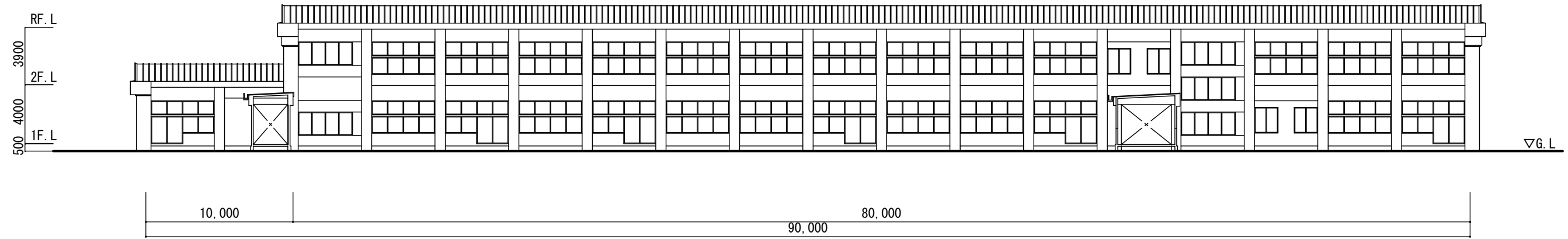
北校舎 南側立面図
