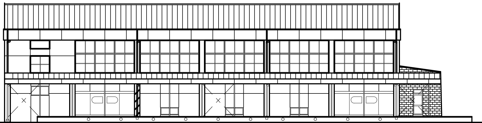
南側立面図
