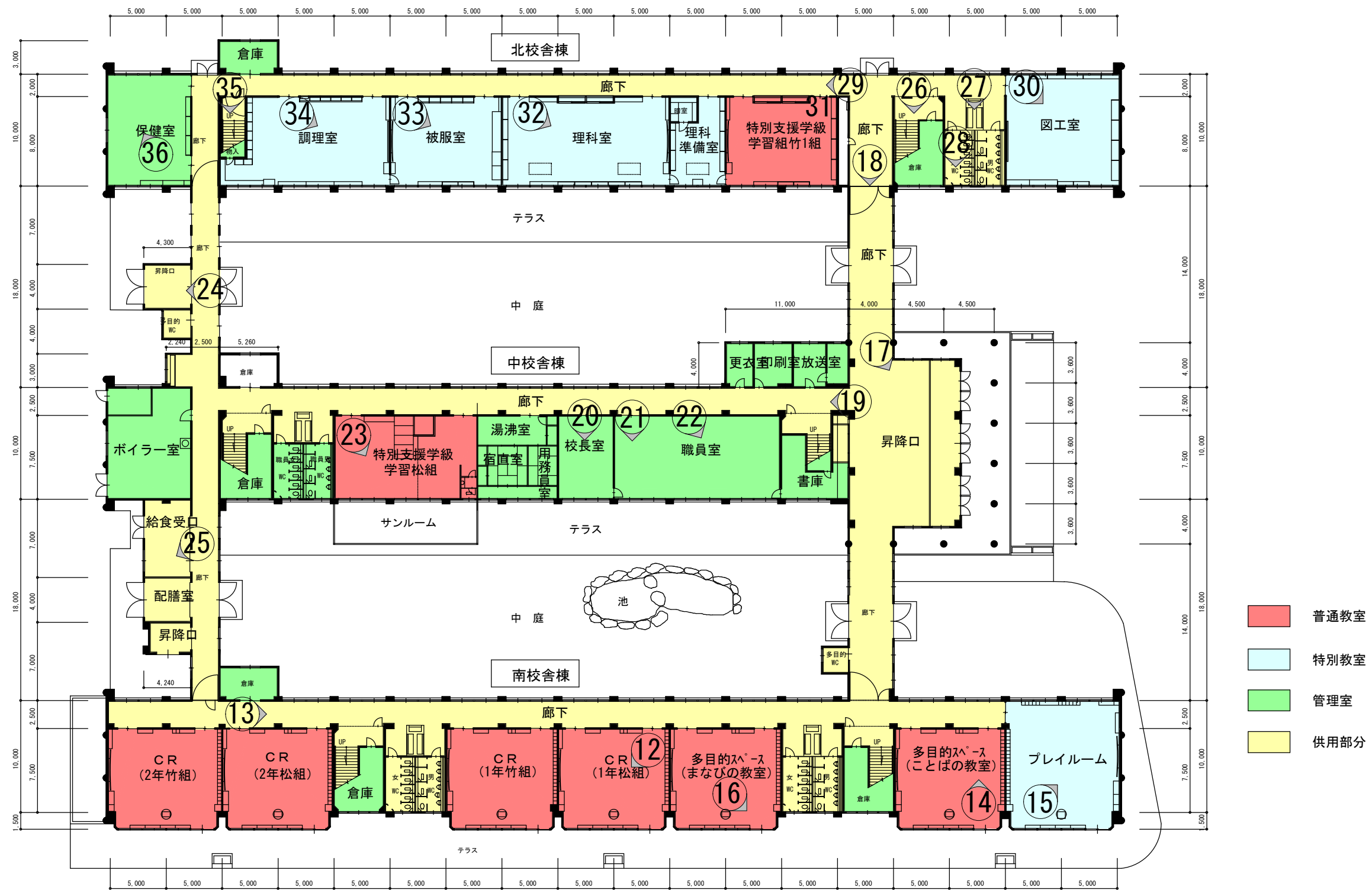
1 階 平 面 図
