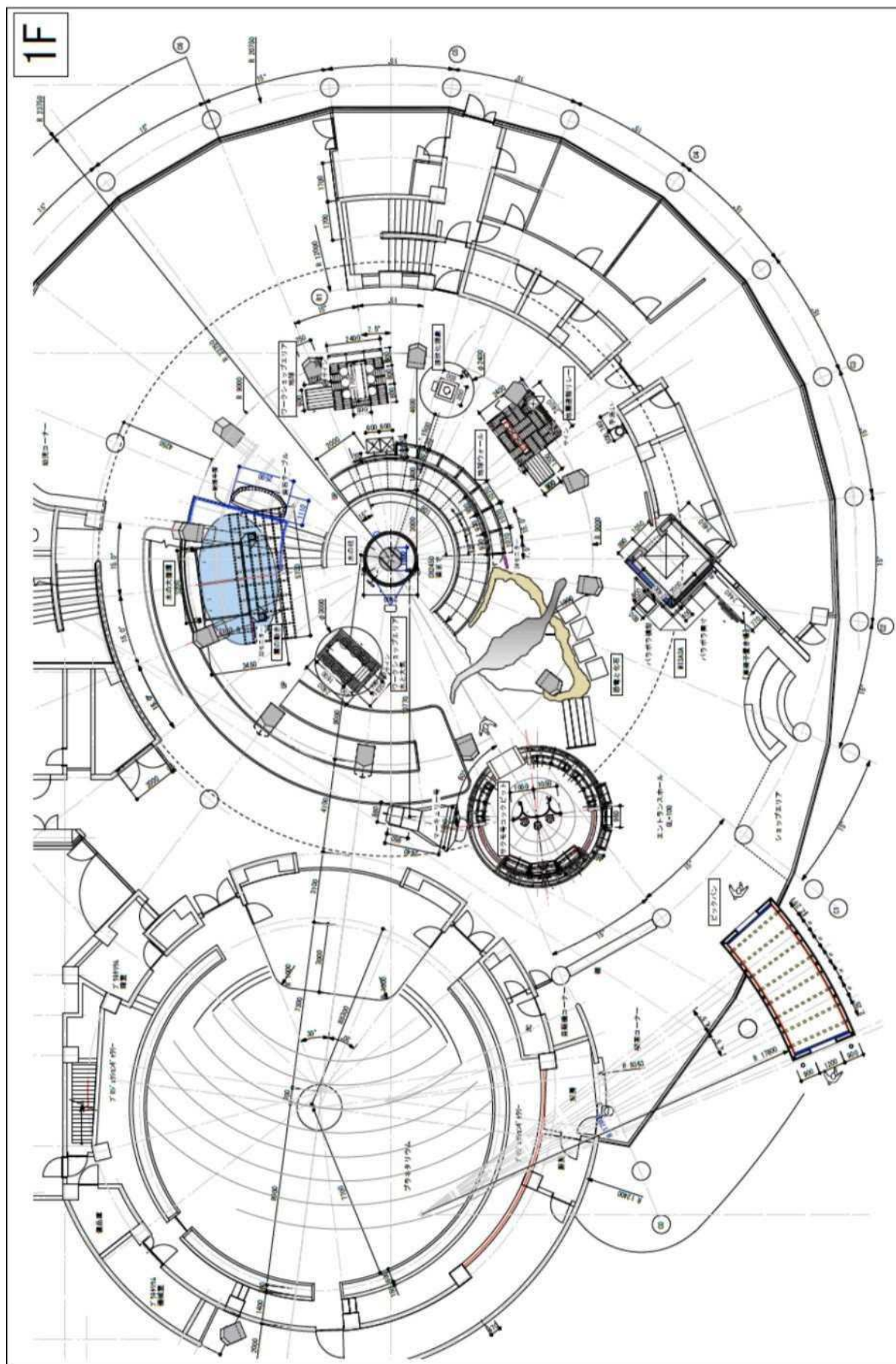
1 階平面図
