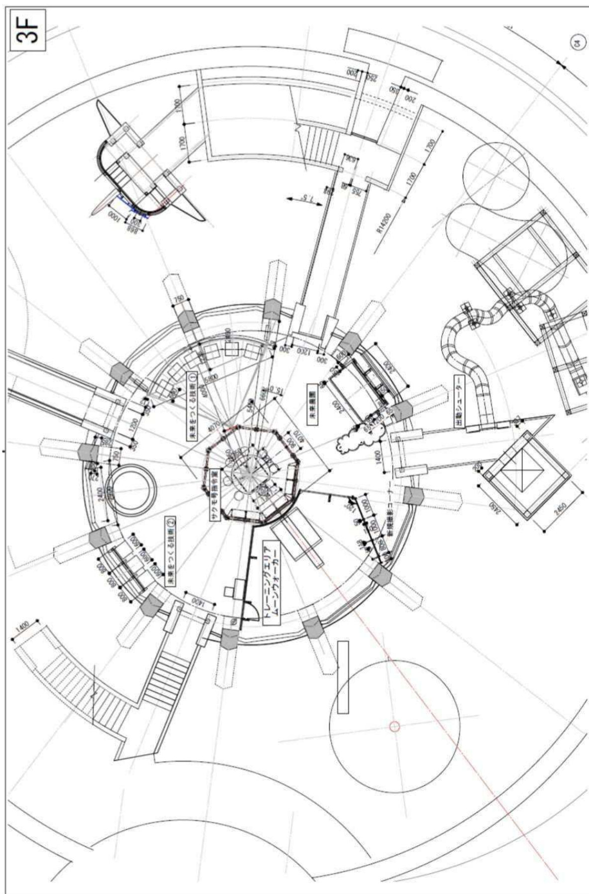
3 階平面図
