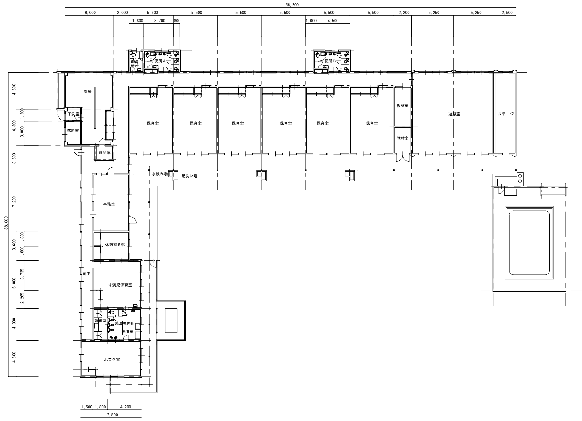
平面図 S = 1/200
