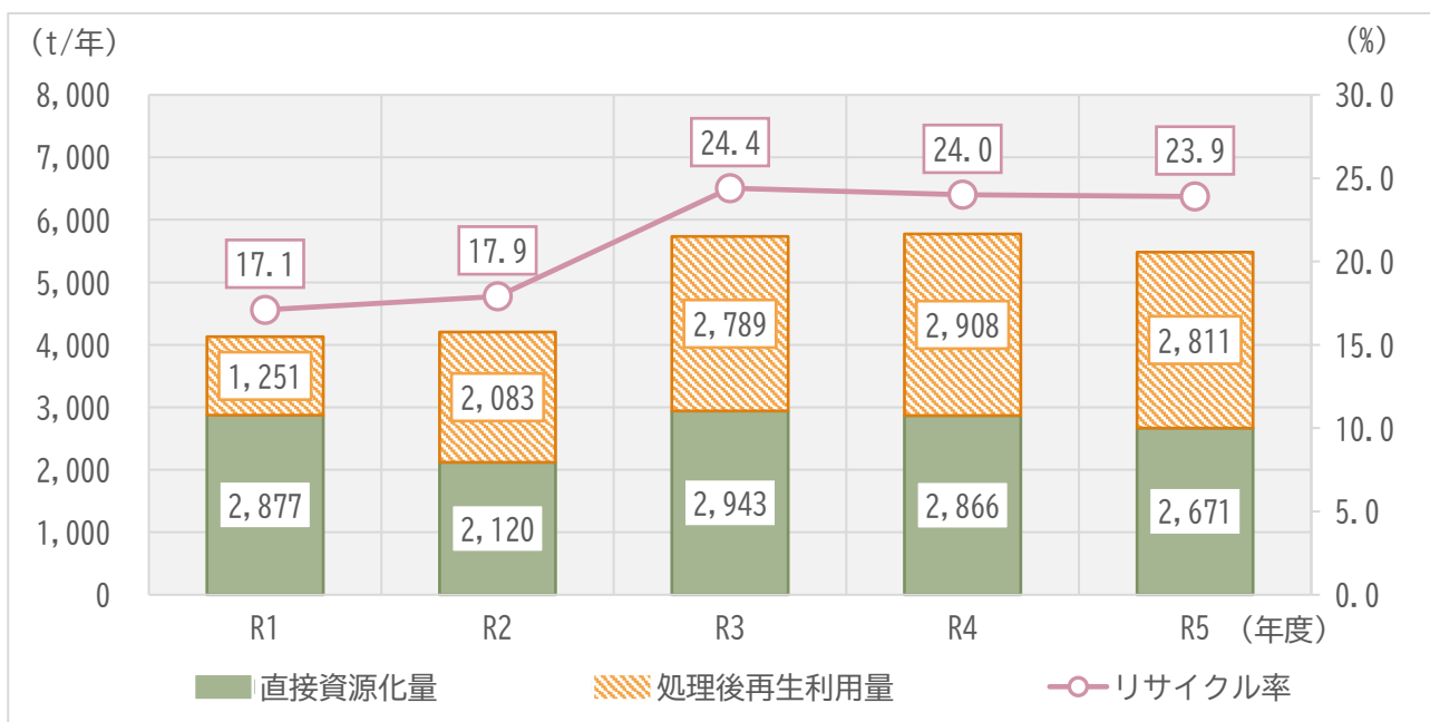
図5 資源化量及びリサイクル率の推移
