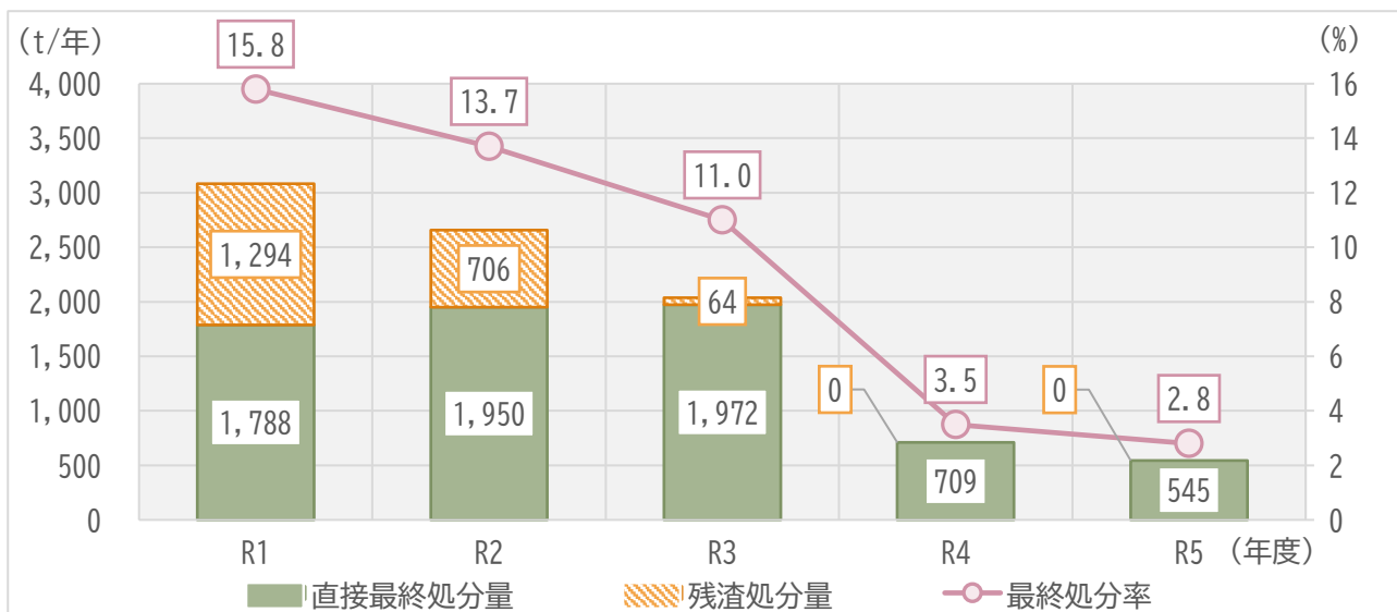
図4 最終処分量及び最終処分率の推移
