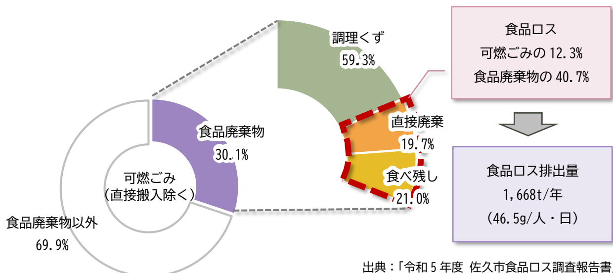
図8 可燃ごみに占める食品ロスの割合と食品ロス排出量（令和4年度）
