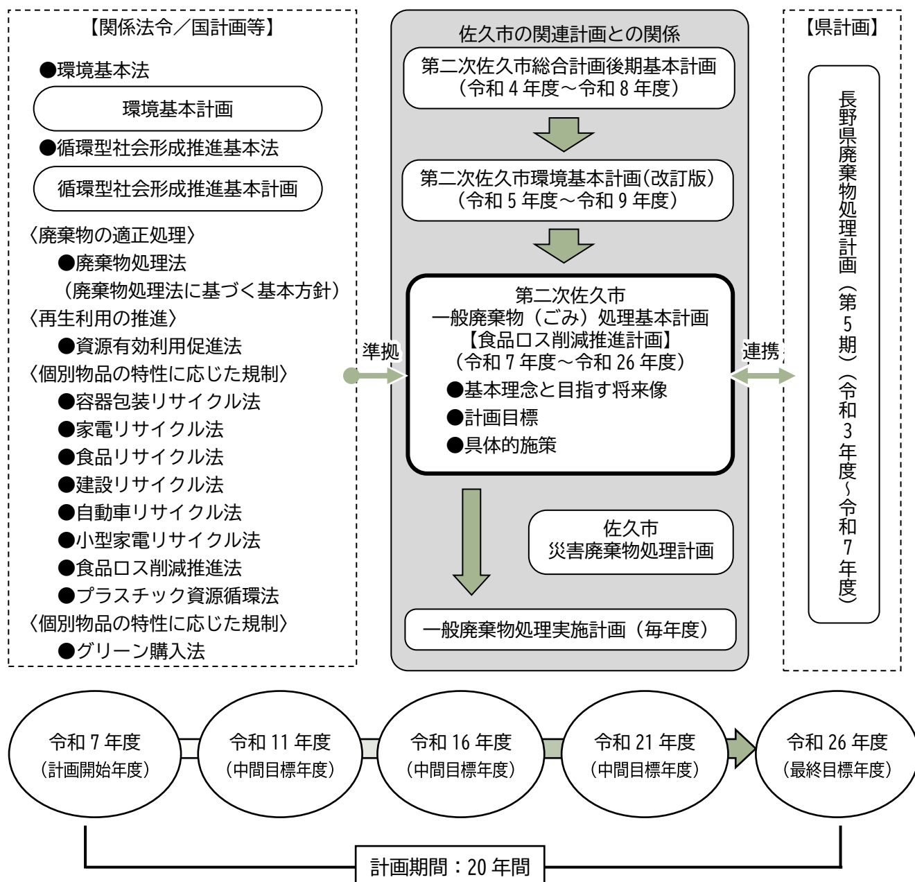
図 1 計画の位置付けと計画期間
