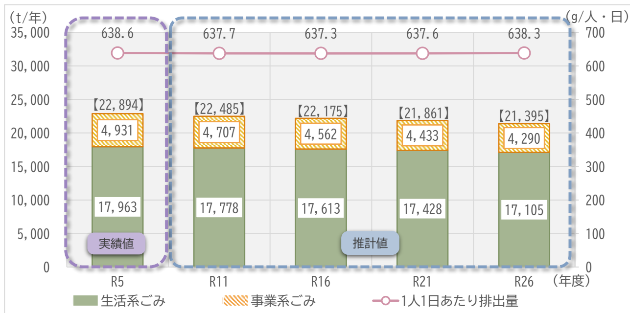
図6 ごみ排出量の推移（現状推移）
