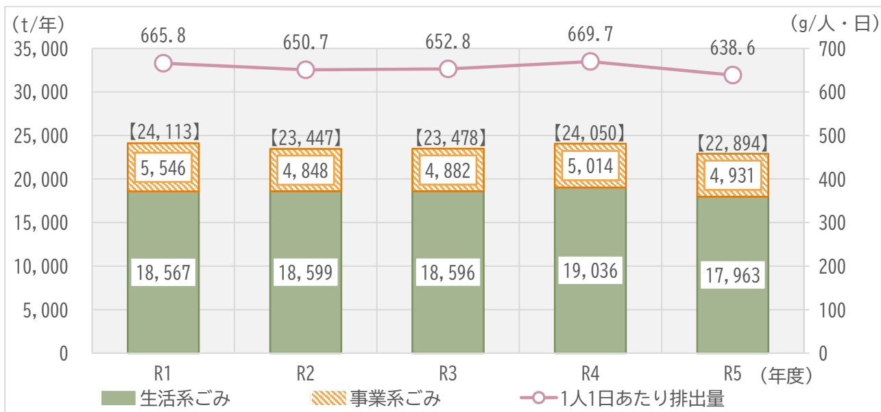
図2 排出源別排出量の推移
