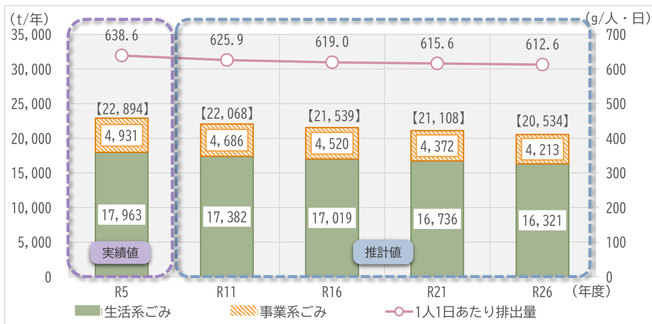
図7 ごみ排出量の推移（目標達成ケース）
