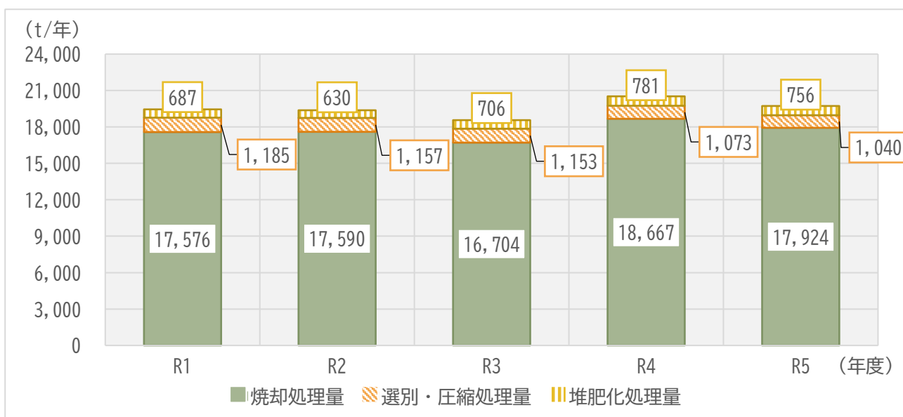
図3 ごみ処理量の推移
