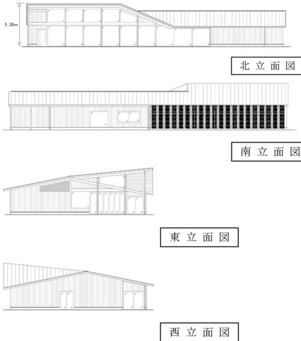
交流施設 立面図
