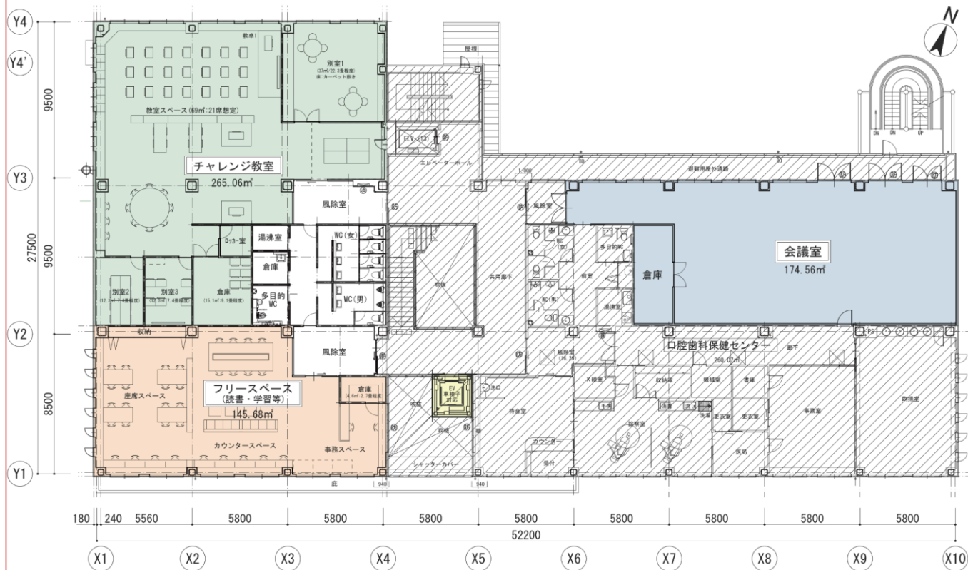
2階平面図
