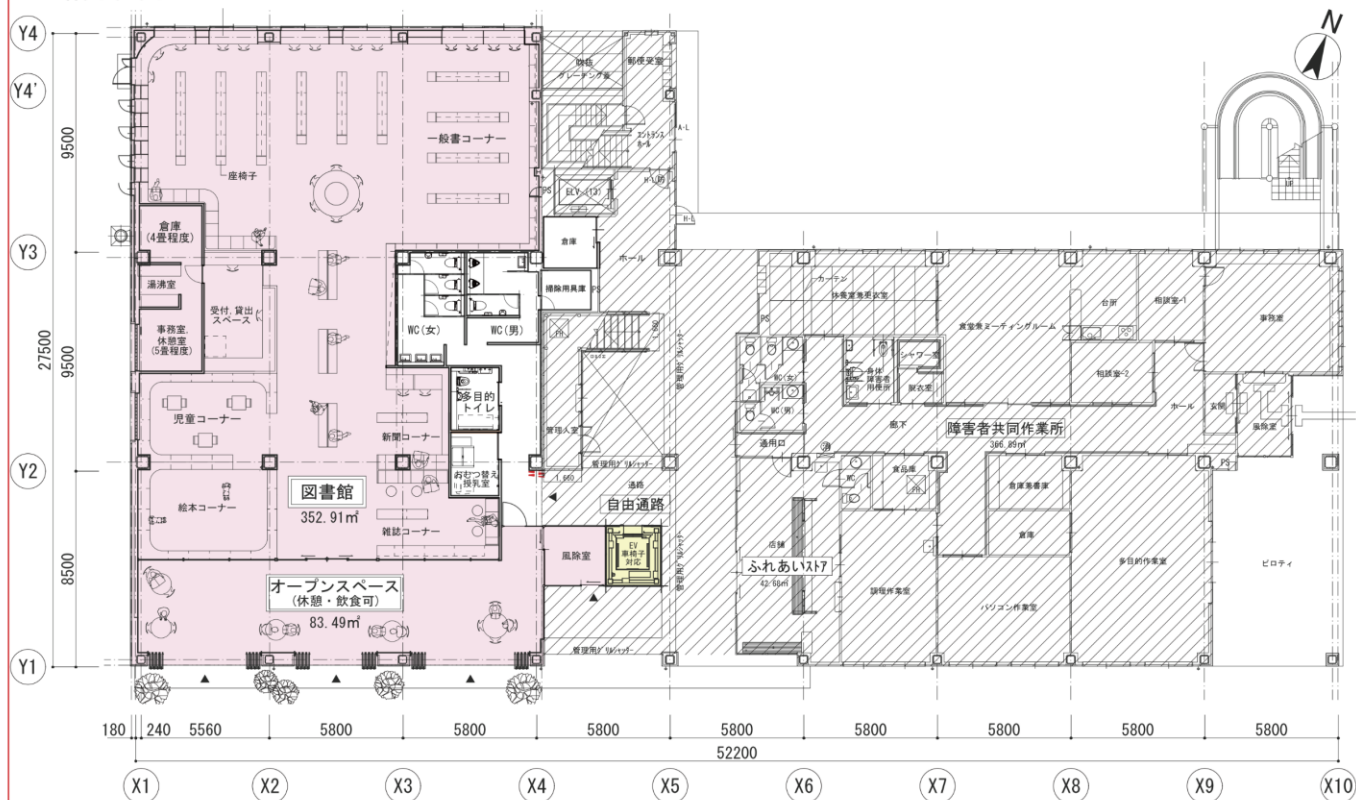
1階平面図
