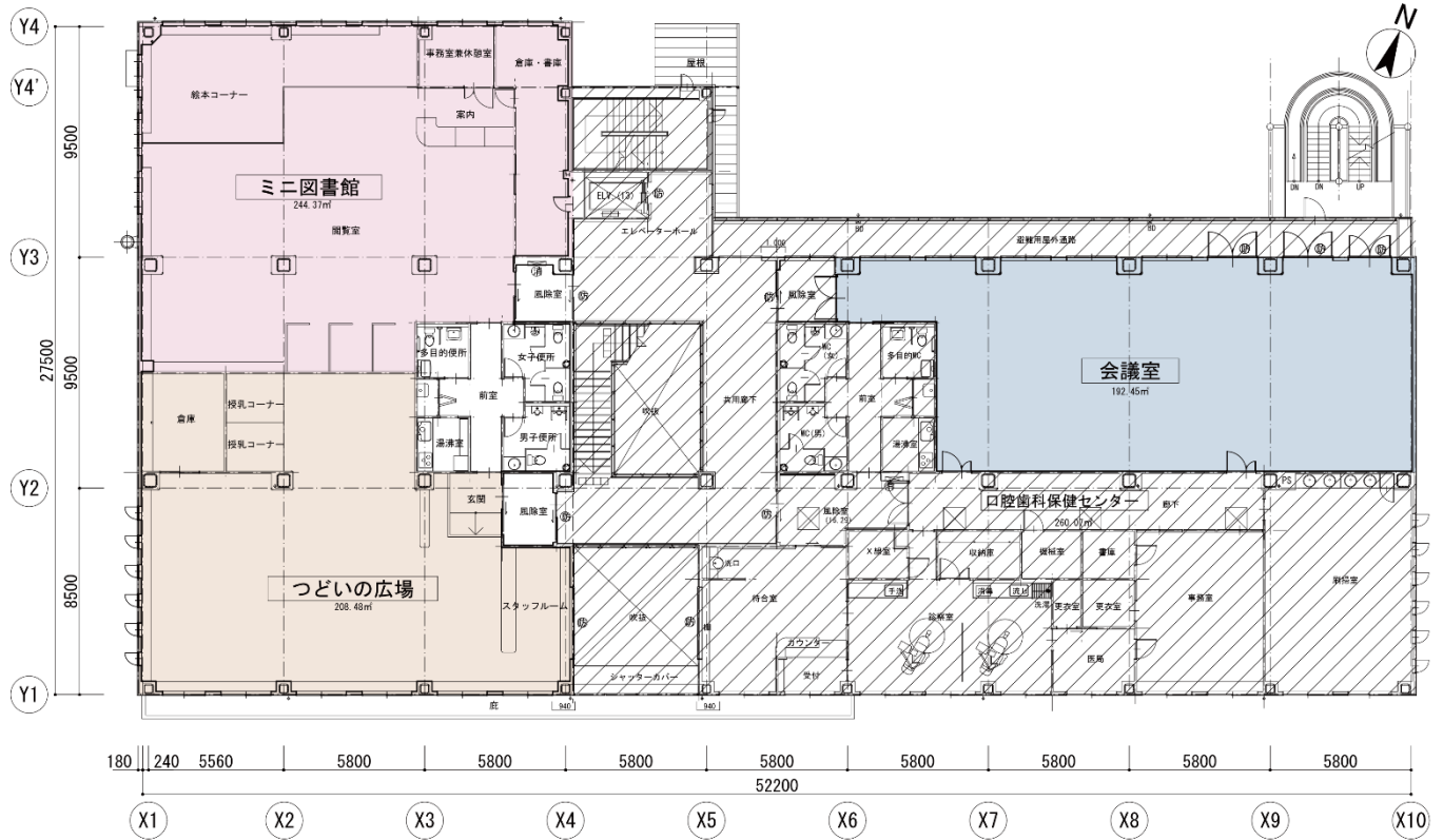
2階平面図
